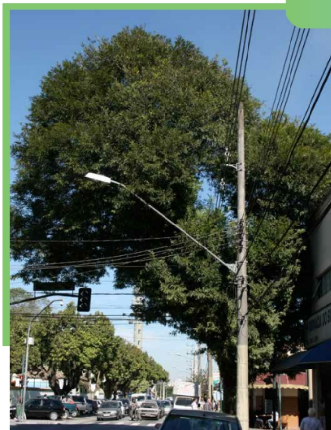
Figura 39 – Área de poda com passagem de rede compacta
