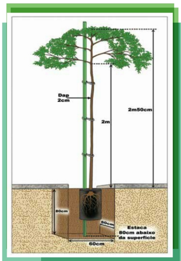
Figura 27 – Plantio de muda padrão e dimensões de cova
